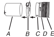
A. Raccord B. Bride de fixation C. Raccord d'évacuation D. Bride de fixation E. Conduit métallique rigide ou souple
